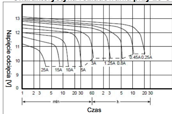
Charakterystyka rozładowania przy 25°C
